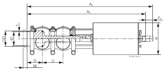
Распределительный клапан
