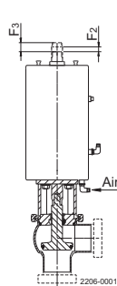
Válvula de cierre con recorrido de dos pasos activada
